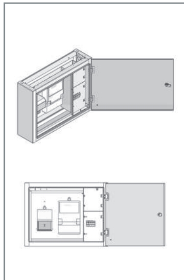
RE 21 M (dvě elektroměrová místa)
